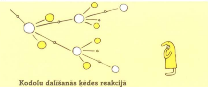
Kodolu dalīšanās ķēdes reakcija
